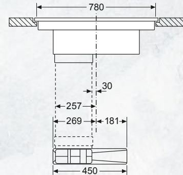
Maße in mm Vorderansicht
