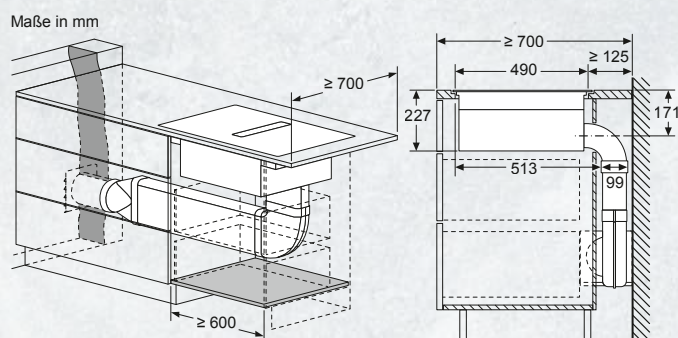
Beispiel Abluft-Führung, Wand
