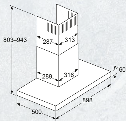
Maße in mm Wandinstallation mit Kamin
