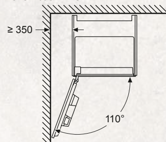
Maße in mm Eckeinbau links
