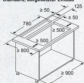
Maße in mm Kombination mit Elektrokochofeld Standard, aufgesetzter Einbau
