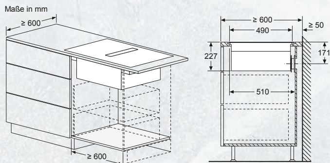
Umluft, ungeführt, Wand
