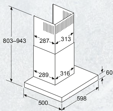
Maße in mm Wandinstallation mit Kamin
