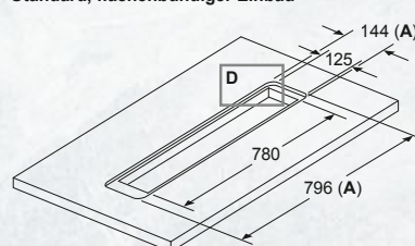
Maße in mm Standard, flächenbündiger Einbau
