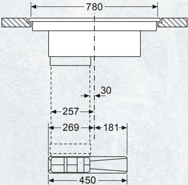
Maße in mm Vorderansicht
