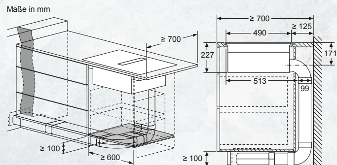
Beispiel geführte Umluft, Wand
