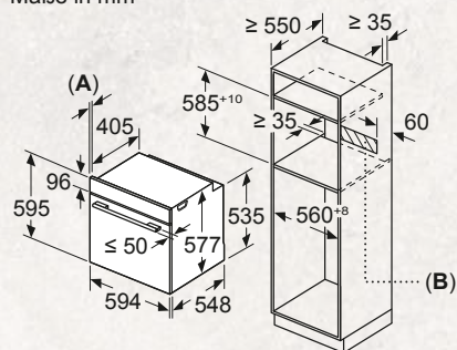
A: 19,5 mm B: Platz für Geräteanschluss 320 x 115 mm
