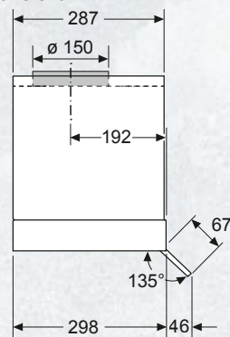
Maße in mm Seitenansicht
