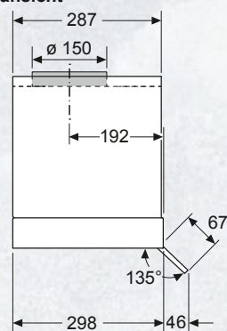
Maße in mm Seitenansicht
