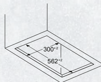
Maße in mm Einbaubeispiel in Möbelausschnitt
