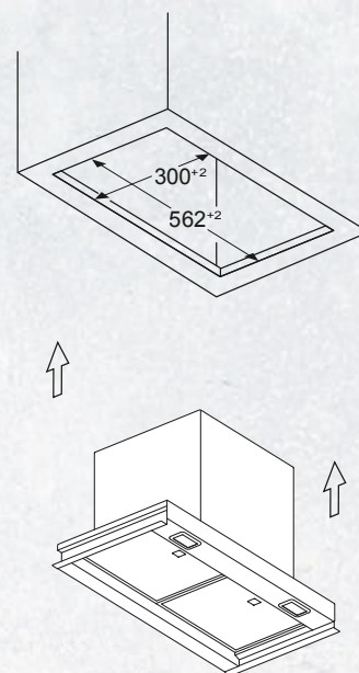
Maße in mm Einbaubeispiel in Möbelausschnitt
