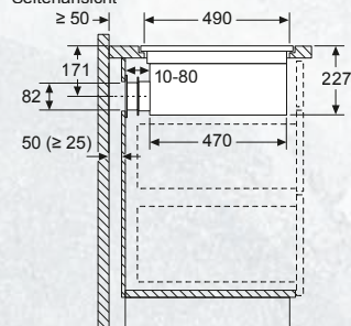
Maße in mm Seitenansicht
