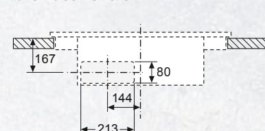
Maße in mm Vorderansicht - Möbelausschnitt für Umluft ohne Kanal
