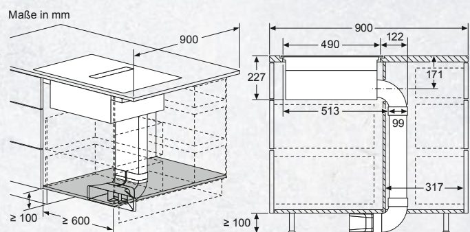
Umluft, teilgeführt, Kochinsel
