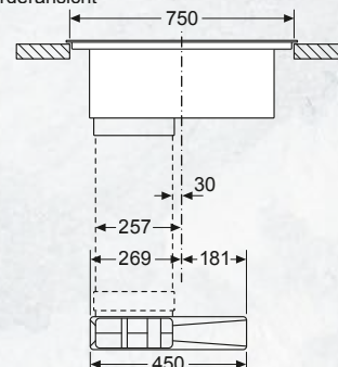
Maße in mm Vorderansicht
