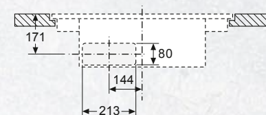
Maße in mm Vorderansicht – Geräteausschnitt für ungesasste Umluft
