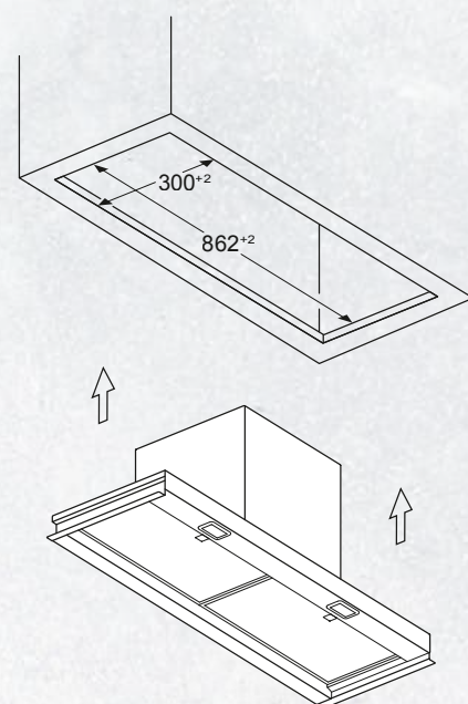
Maße in mm Einbaubeispiel in Möbelausschnitt
