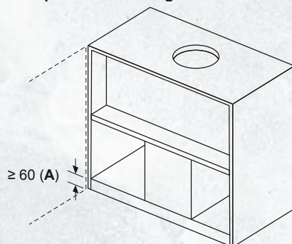
Maße in mm Einbaubeispiel mit Gewürzregal
