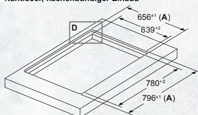
Maße in mm Kombination mit Elektrokochofeld Nahtloser, flächenbündiger Einbau
