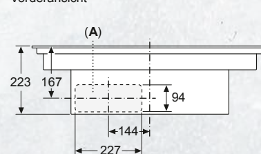
Maße in mm Vorderansicht
