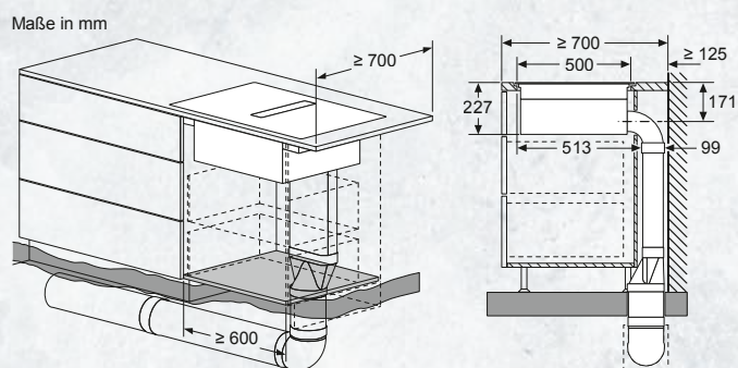
Beispiel Abluft-Führung in den Boden, Wand
