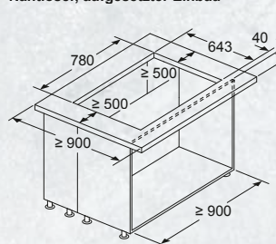
Maße in mm Kombination mit Elektrokochofeld Nahtloser, aufgesetzter Einbau
