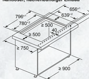
Maße in mm Kombination mit Elektrokochofeld Nahtloser, flächenbündiger Einbau
