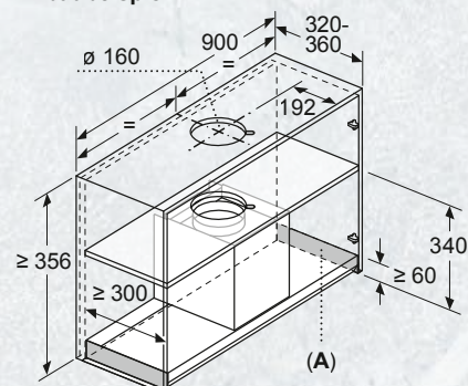
Maße in mm Einbaubeispiel
