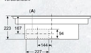
Maße in mm Vorderansicht
