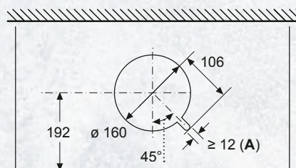
Maße in mm Ansicht von oben
