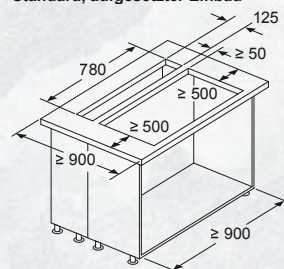
Maße in mm Kombination mit Elektrokochofeld Standard, aufgesetzter Einbau
