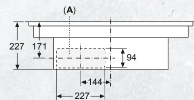
Maße in mm Vorderansicht
