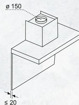
Maße in mm Wandblendentiefe
