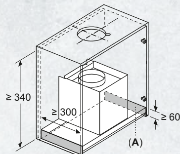
Maße in mm Installationsanforderungen für den Ersatzbedarf
