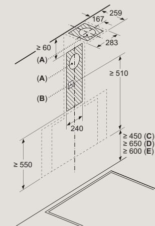
Wandinstallation mit Kamin
