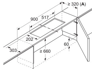
Montage Flachschräume mit Clean Air Modul und Absenkrahmen
