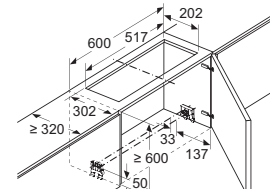
Montage Flachschräume mit Umluftset
