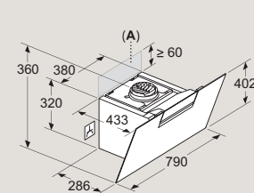
Gerät im Umluftbetrieb ohne Abluftkanal
