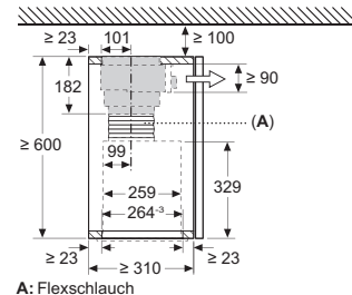
Montage Lüfterbaustein mit Umluftset
