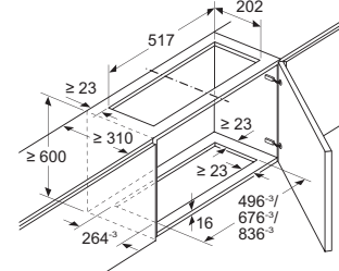
Montage Lüfterbaustein mit Umluftset
