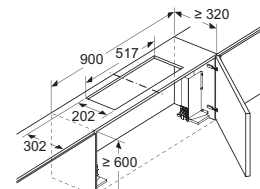
Montage Flachschräume mit Umluftset
