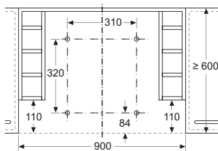
Montage Flachschrühube mit Absenkrahmen Möbel mit seitlichen Regalfächern Montage direkt an der Küchenwand
