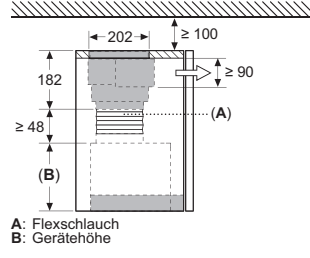
Montage integrierte Designhaube mit einem Umluftset
