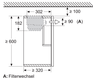
Montage Flachschräume mit Umluftset
