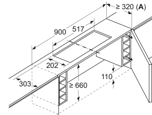
Montage Flachschräume mit Clean Air Modul und Absenkrahmen
