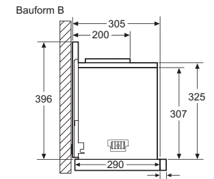
Montage bei Geräten mit Absenkrahmen - Möbelkorpus-tiefe laut Kombinationstabelle
