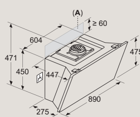
Gerät im Umluftbetrieb ohne Abluftkanal
