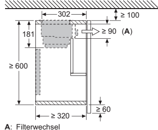
Montage Flachschräume mit Clean Air Modul und Absenkrahmen
