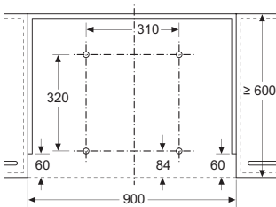
Montage Flachschrühube mit Absenkrahmen Montage direkt an der Küchenwand
