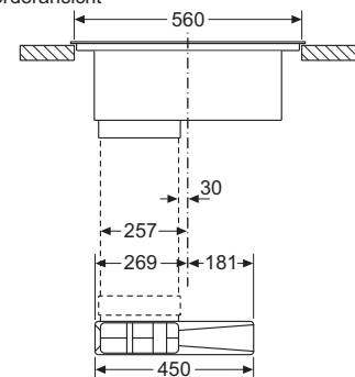
Vorderansicht
