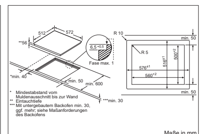
PVS601FB5E – flächenbündig
