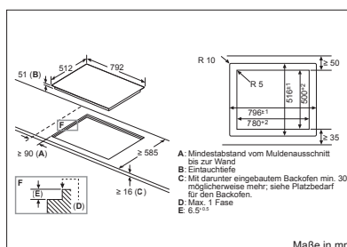
PKM801DP2D – flächenbündig
