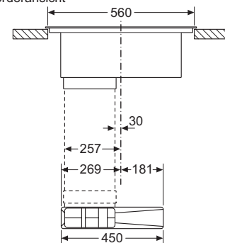
Vorderansicht
