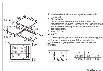
PXV821DV5E – flächenbündig
