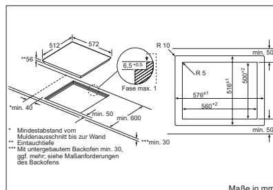
PXY621DX6E – flächenbündig
