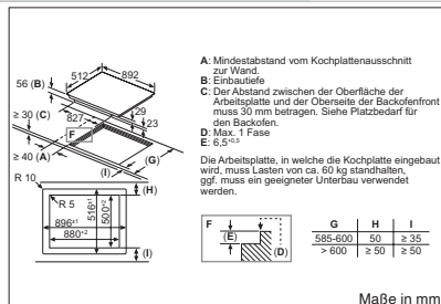
PXX921DX6E – flächenbündig
