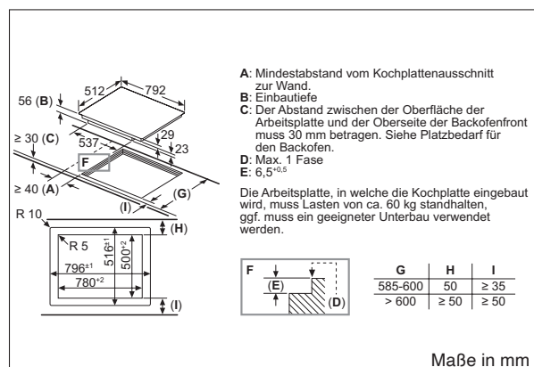
PXY828DX6E – flächenbündig
