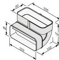
Flachkanalbogen DFK-BVK 90
