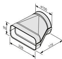
Flachkanaladapter DFK-A
