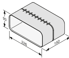
Längenausgleichsleiste Flachkanal DFK-L
