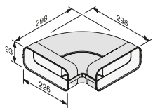
Flachkanalbogen DFK-BH 90
