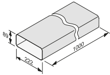
Flachkanal DFK-R 1000
