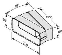
Flachkanalbogen DFK-BH 15
