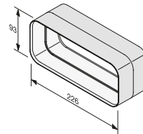
Verbindungsstück Flachkanal DFK-V
