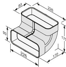
Flachkanalbogen DFK-BV 90
